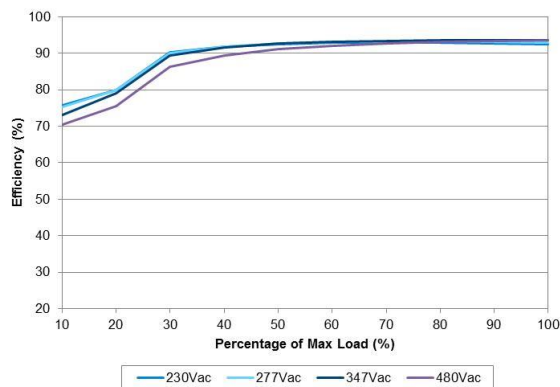
LNV-48V320W□
